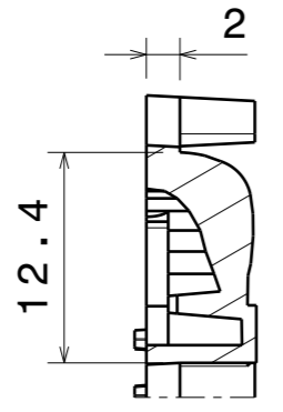
Section view A-A Scale: 2:1
