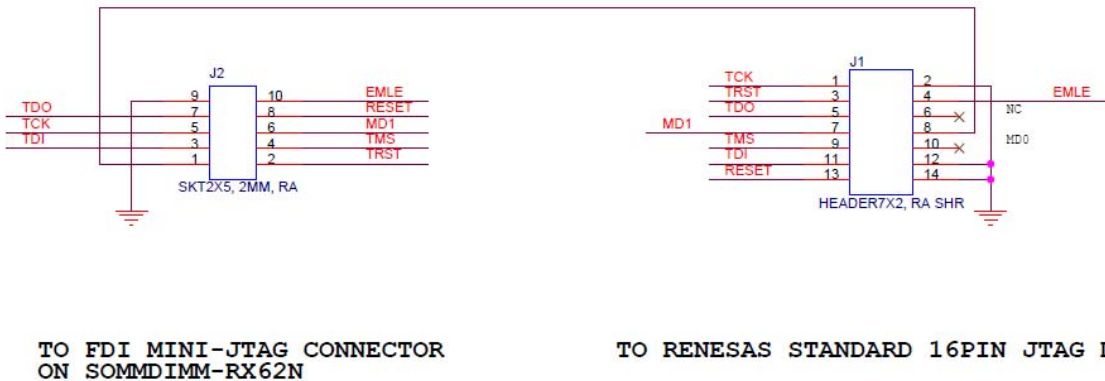
Figure 5 – Mini JTAG Adapter Wiring Diagram
