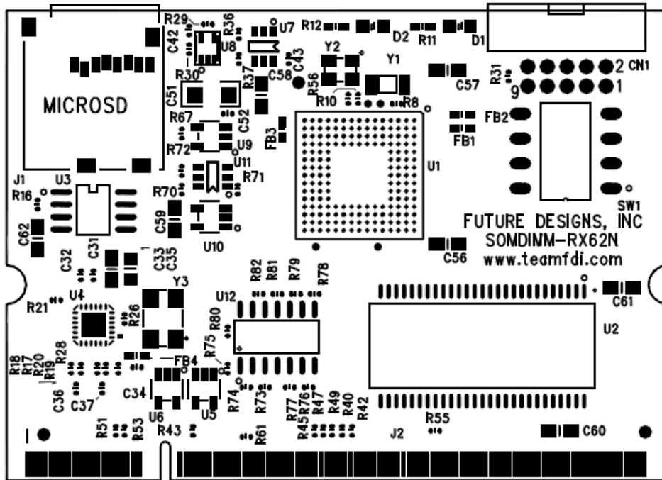
Figure 2 – SOMDIMM-RX62N Side
